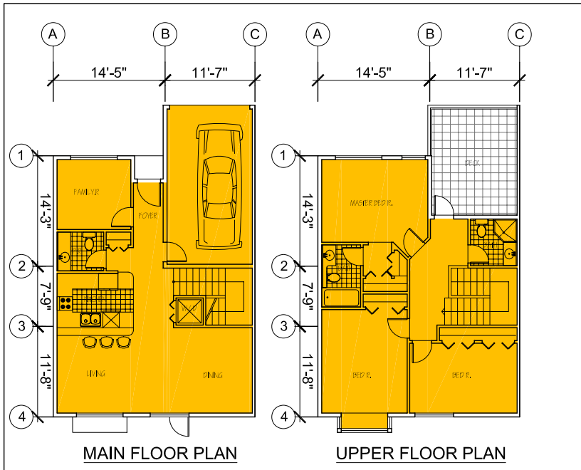
UNIT A SCALE: 1/8
