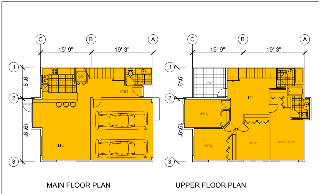
UNIT D SCALE: 1/8
