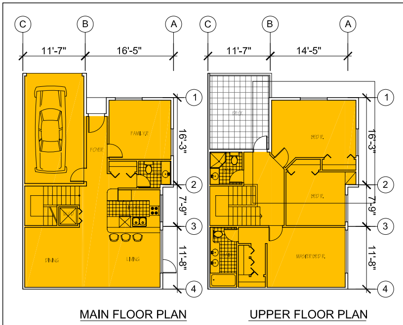
UNIT B SCALE: 1/8
